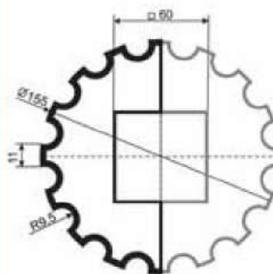
КЛВ-155/1 целая (2000/2500)
