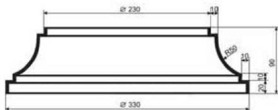
КЛВ-205/1 половина
