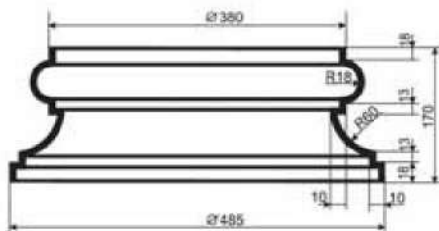
KLIV-355/1 половина
