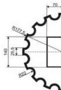
KLIV-355/2 половина (2000/2500)
