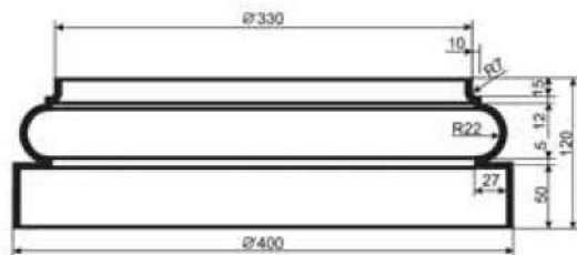
КЛВ-305/1 половина
