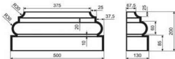
ПЛВ-350/1
