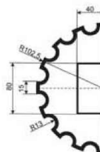
КЛВ-205/2 половина (2000/2500)
